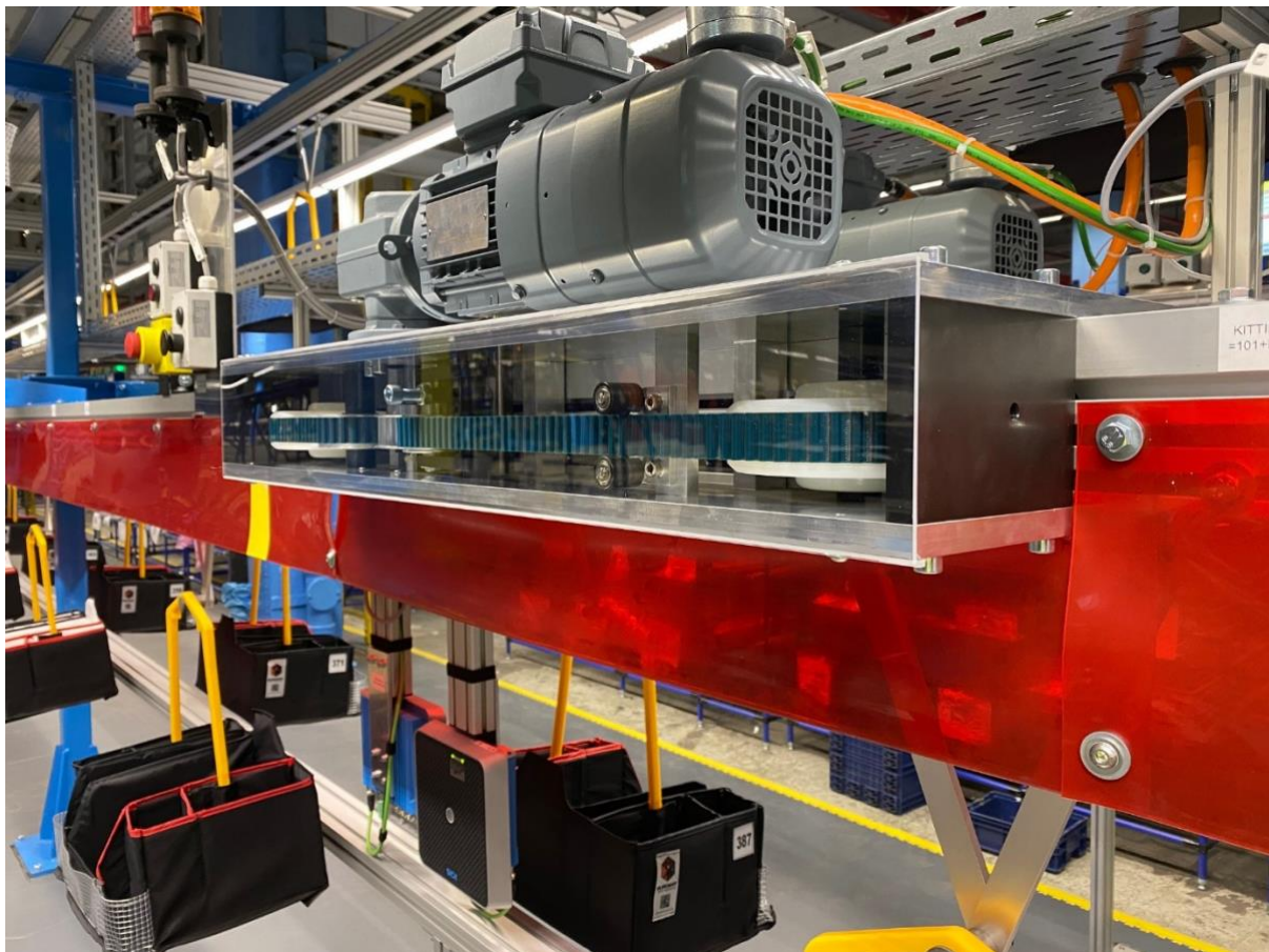
Bild: Kommissionierkörbe an der QuickMOVE Strecke
